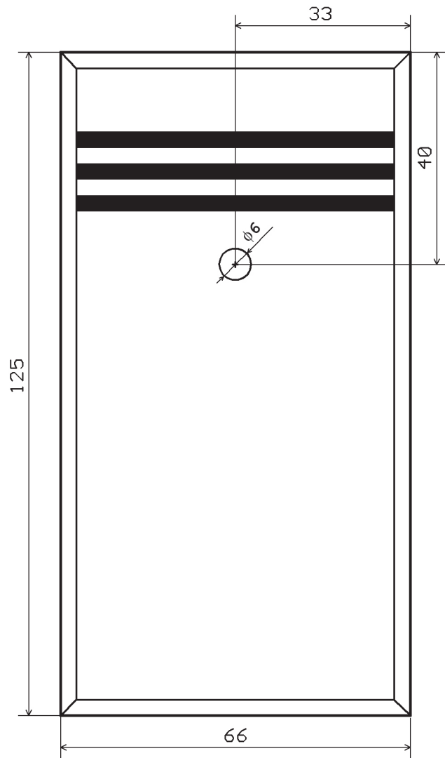
Pohled shora
