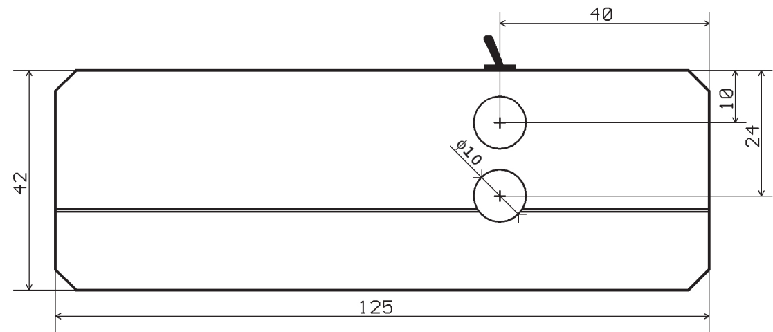
Pohled zprava
